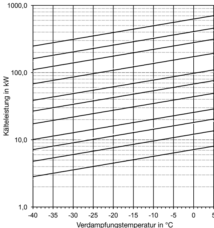
MINIMALE KÄLTELEISTUNG
