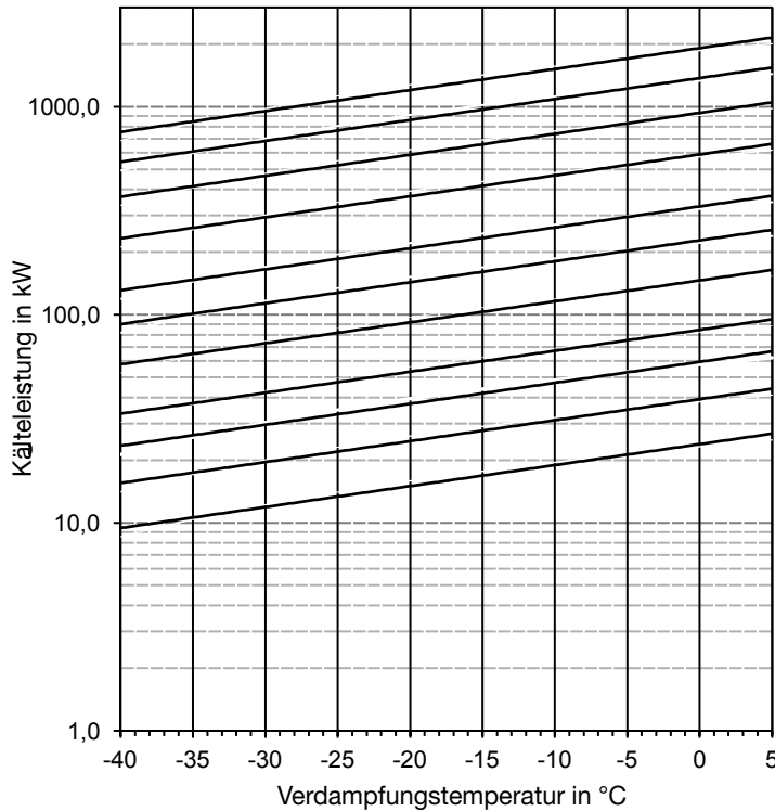
MAXIMALE KÄLTELEISTUNG
