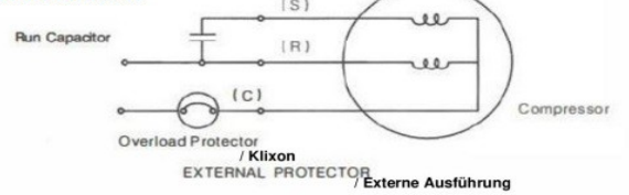
Betriebskondensator
