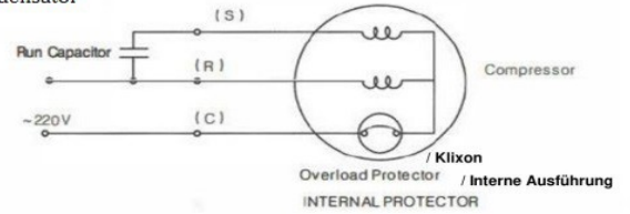
Betriebskondensator
