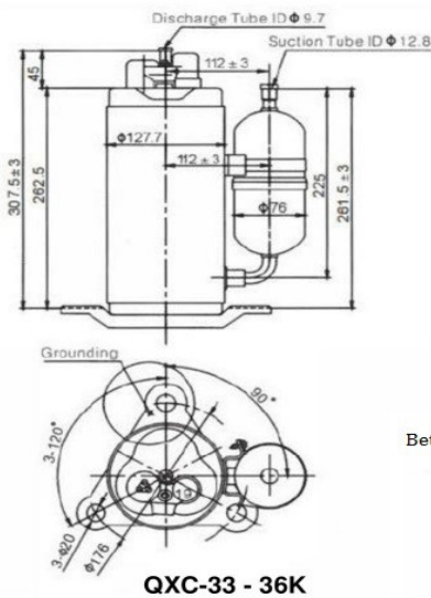
QXC-33 - 36K
