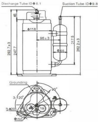
QXC-10 - 16K
