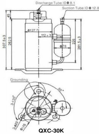
QXC-30K
