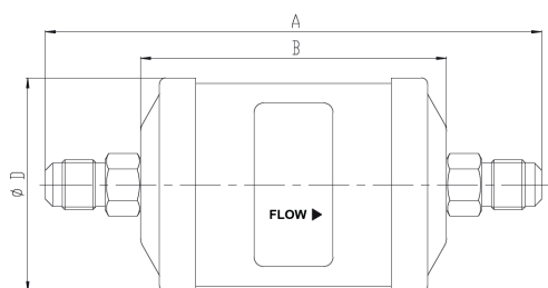
Bördelanschluss
