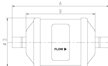
Lötanschluss
